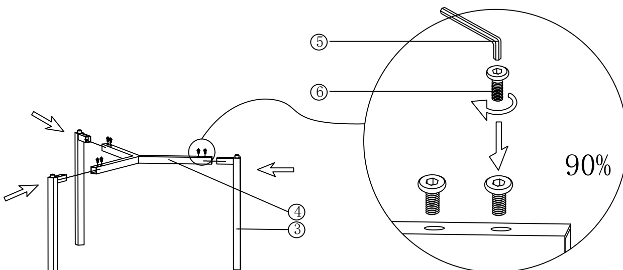
A Lange schroeven gebruiken
