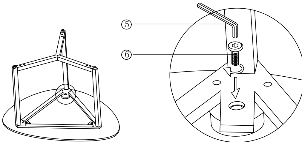
D Korte schroef gebruiken
