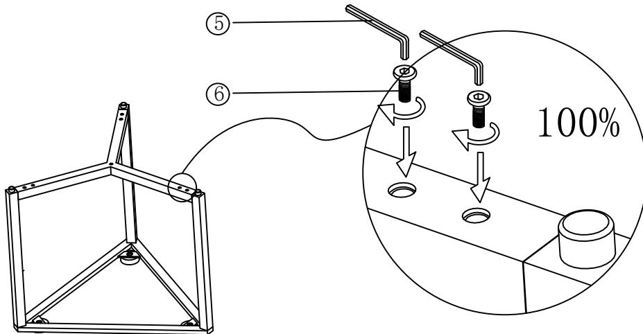
C Lange schroeven gebruiken
